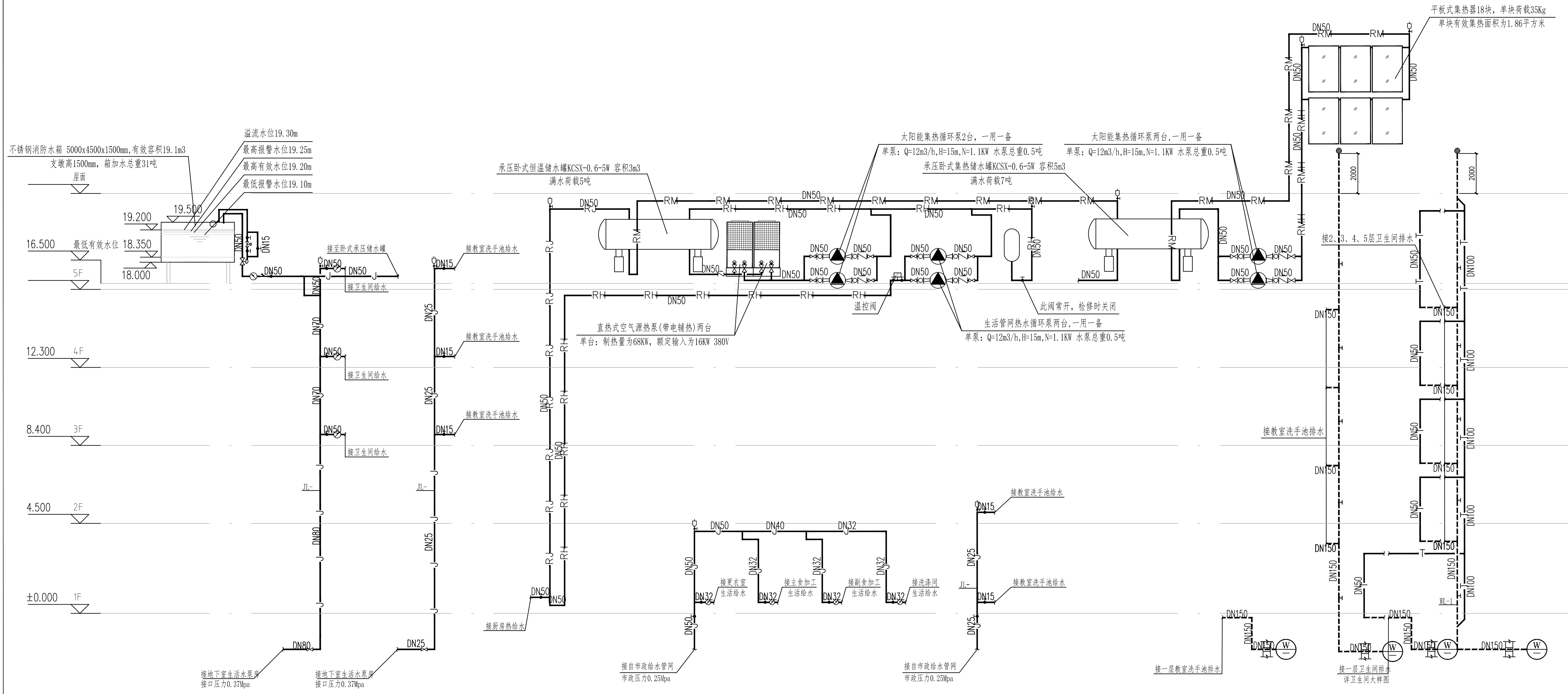
生活给水系统原理图
