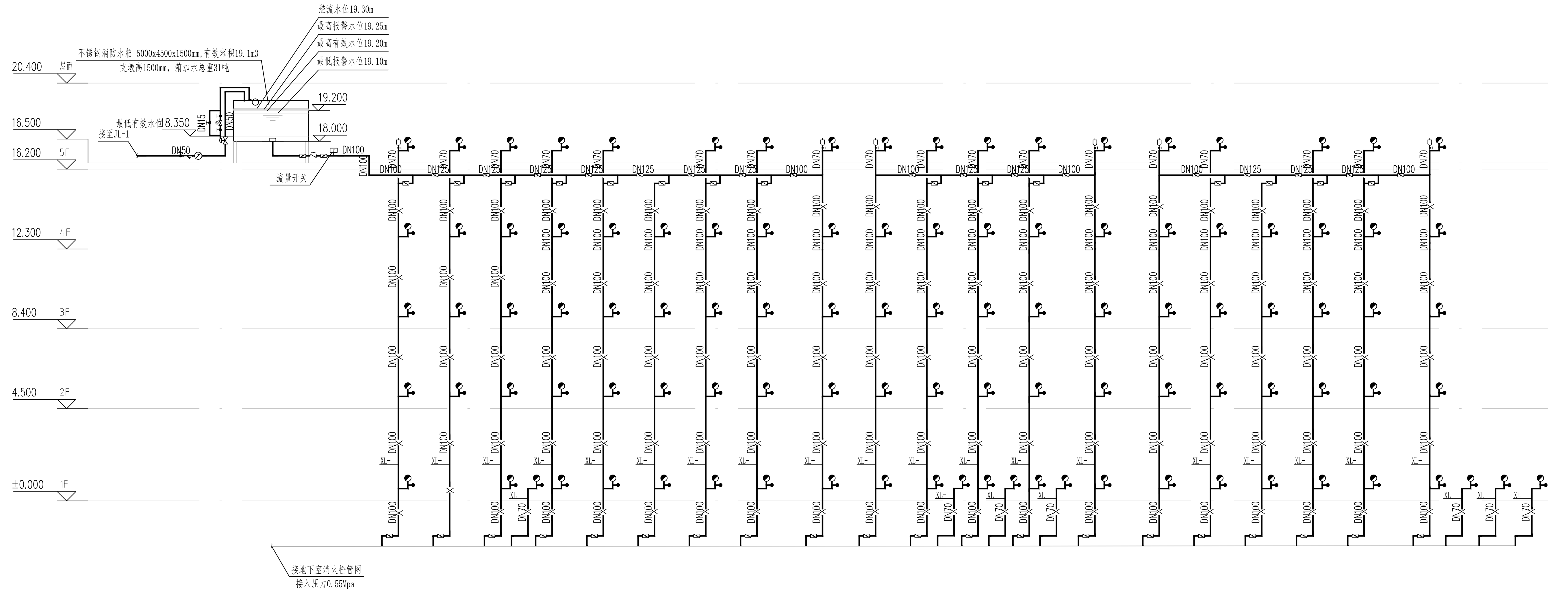
地上室内消火栓系统原理图
