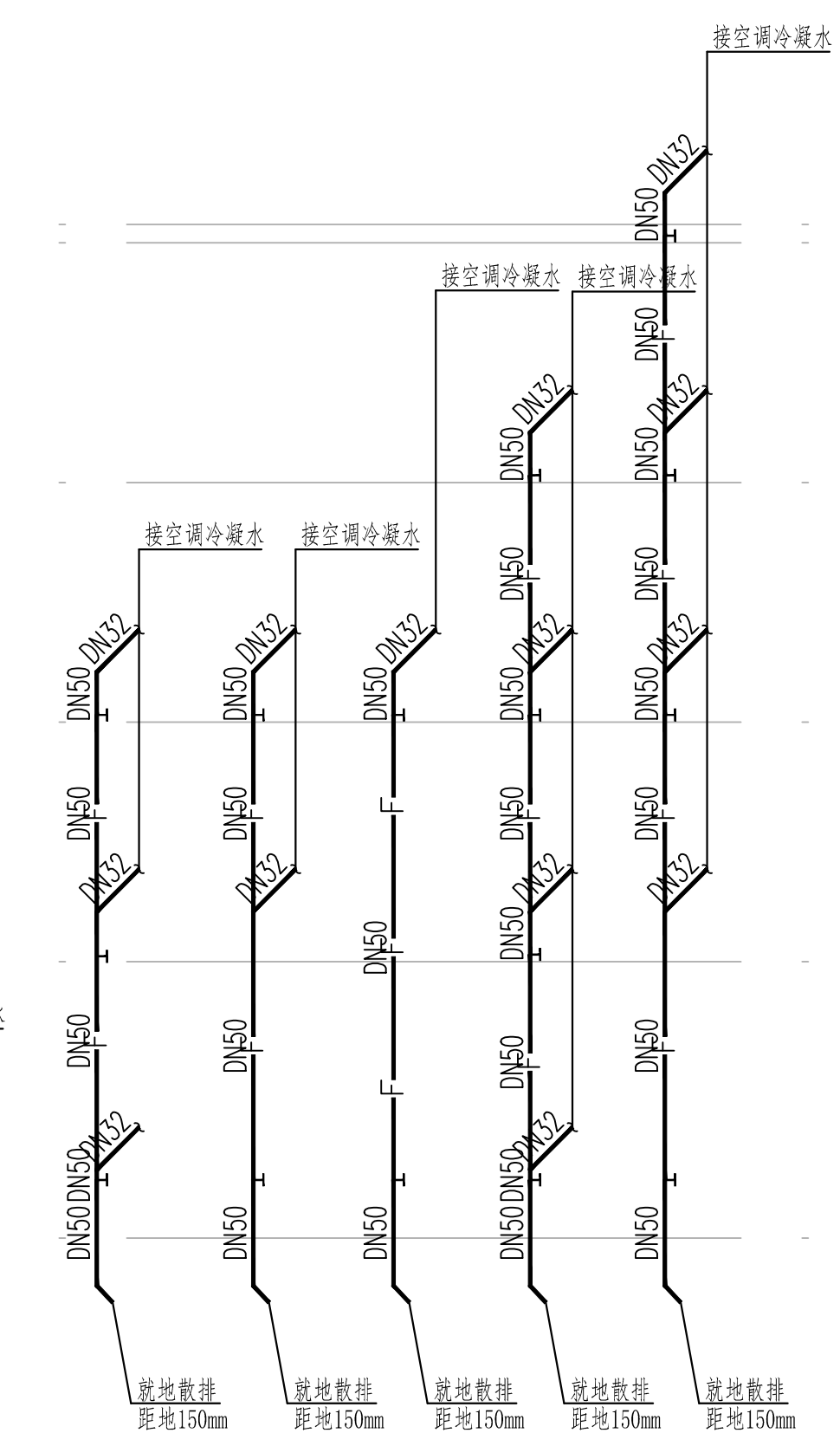
地上空调废水系统原理图
