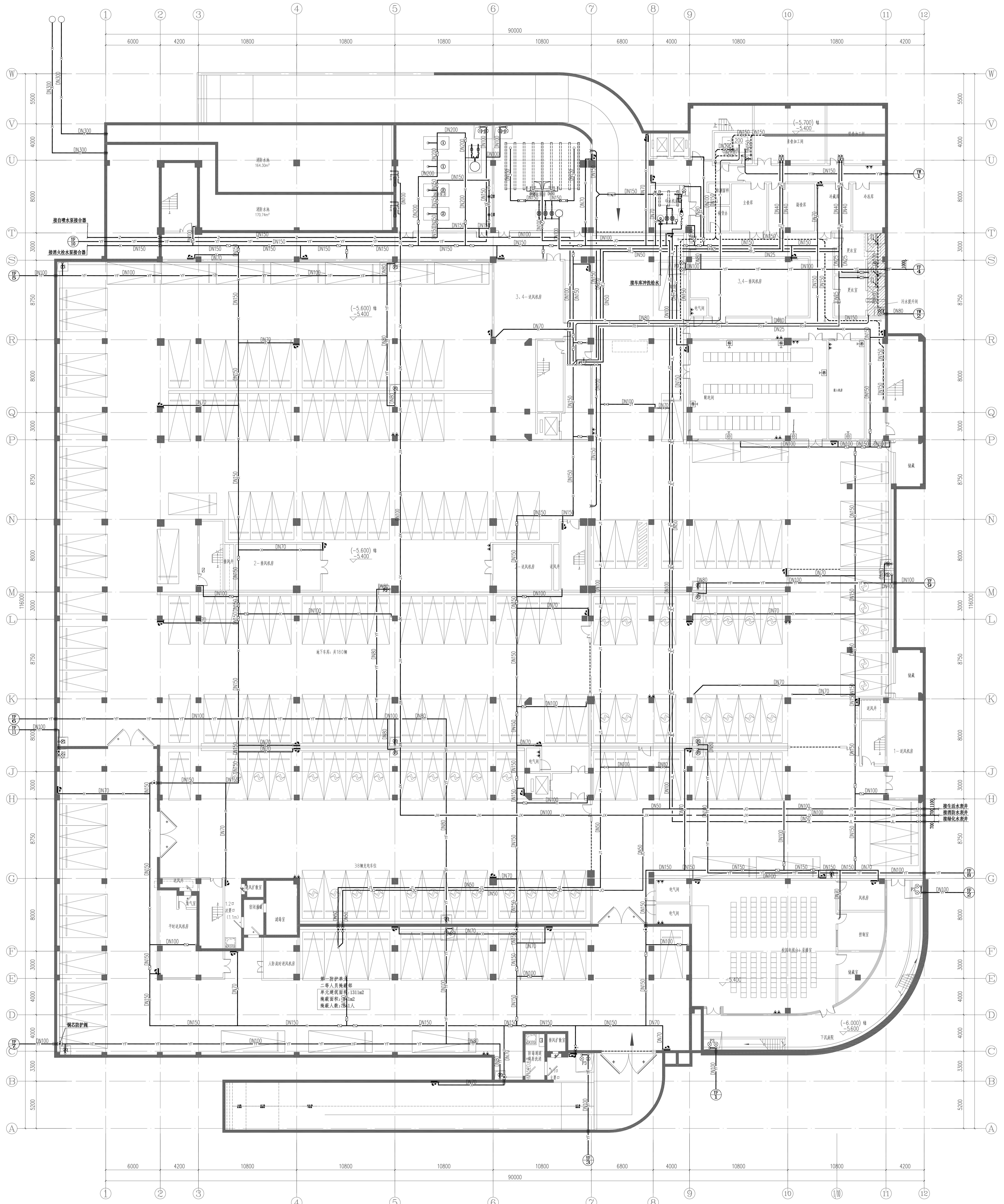
地下室给排水、消火栓平面图 1:150
