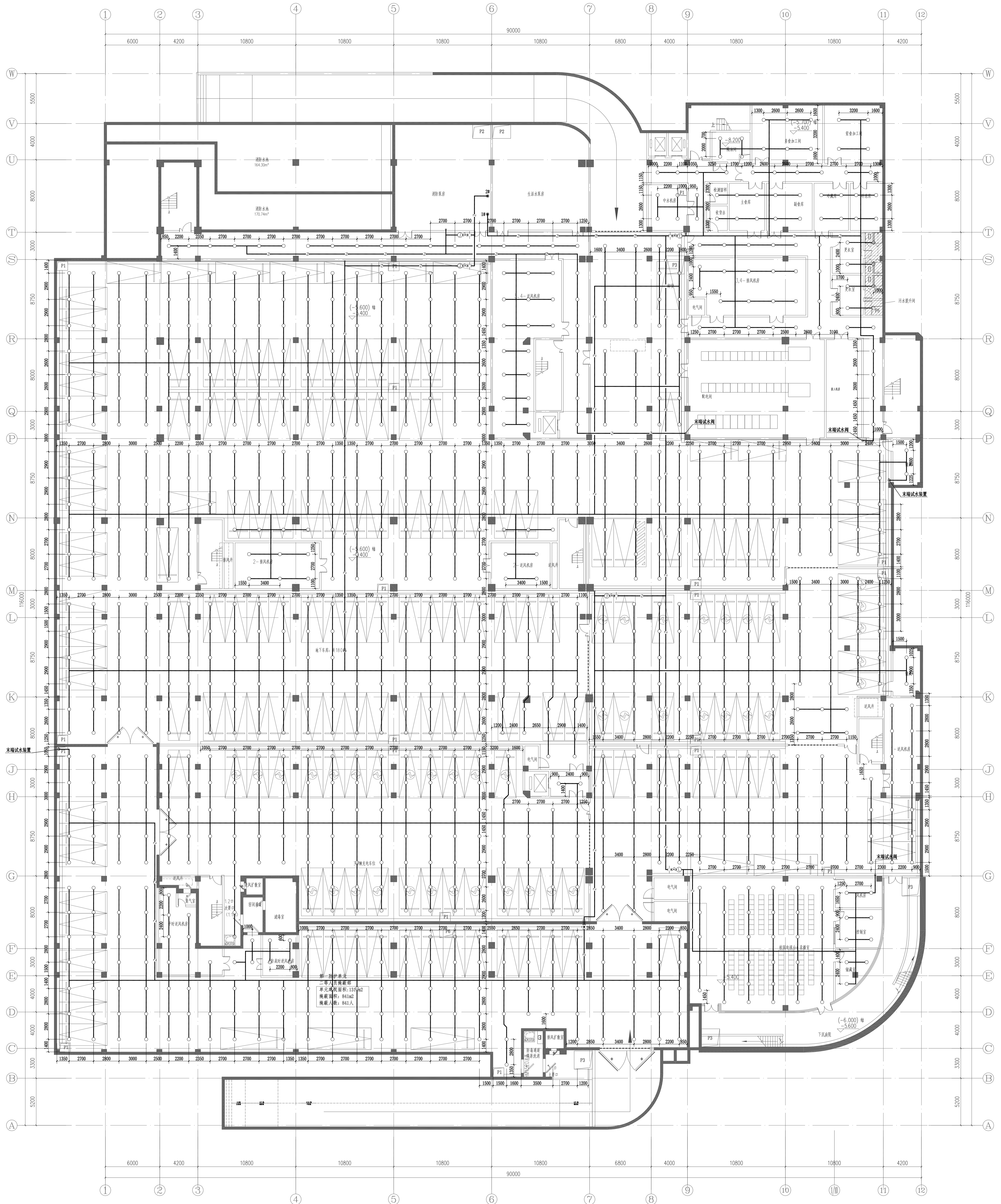
地下室自喷平面图 1:150
