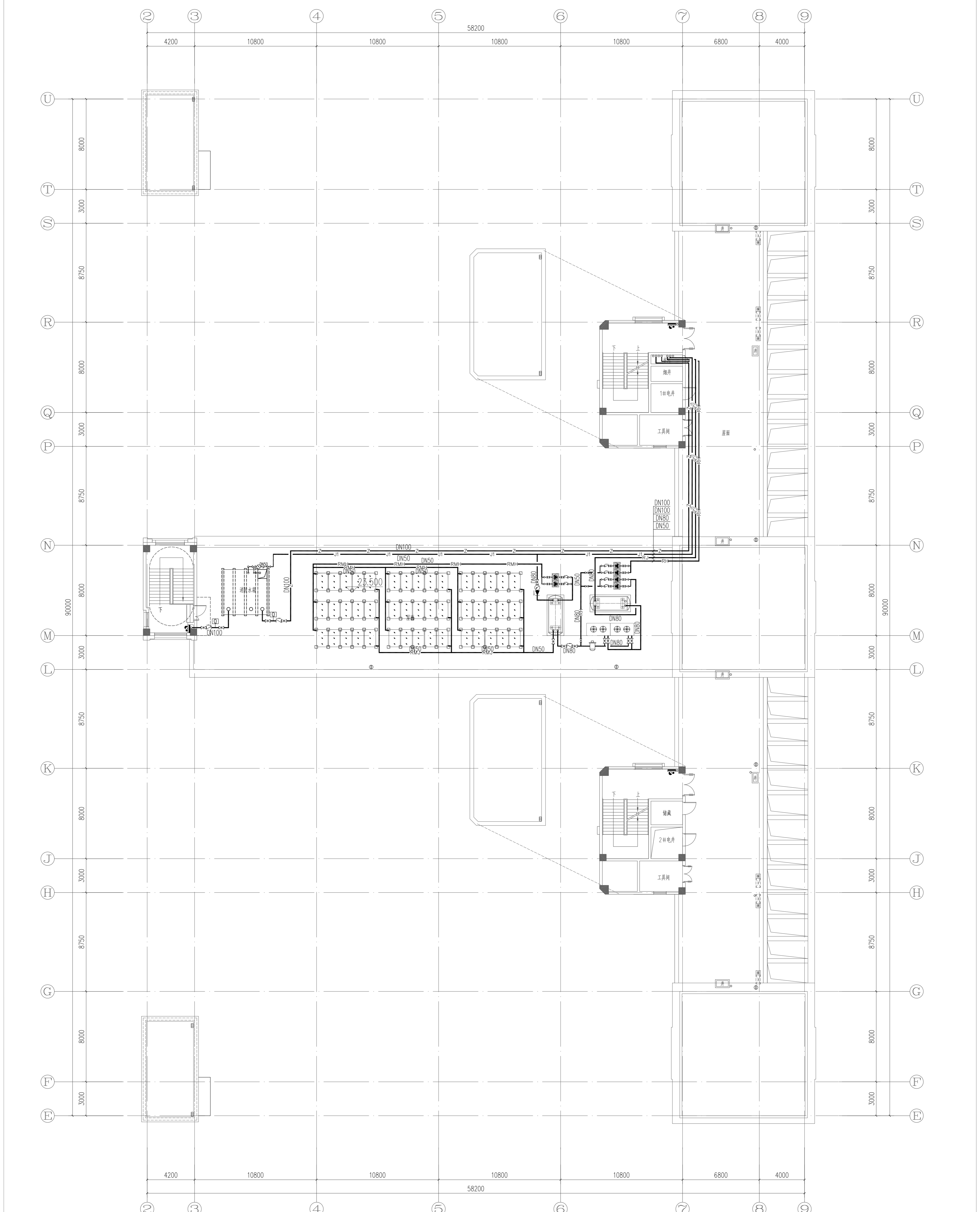
屋面层给排水、消防栓平面图 1:150
