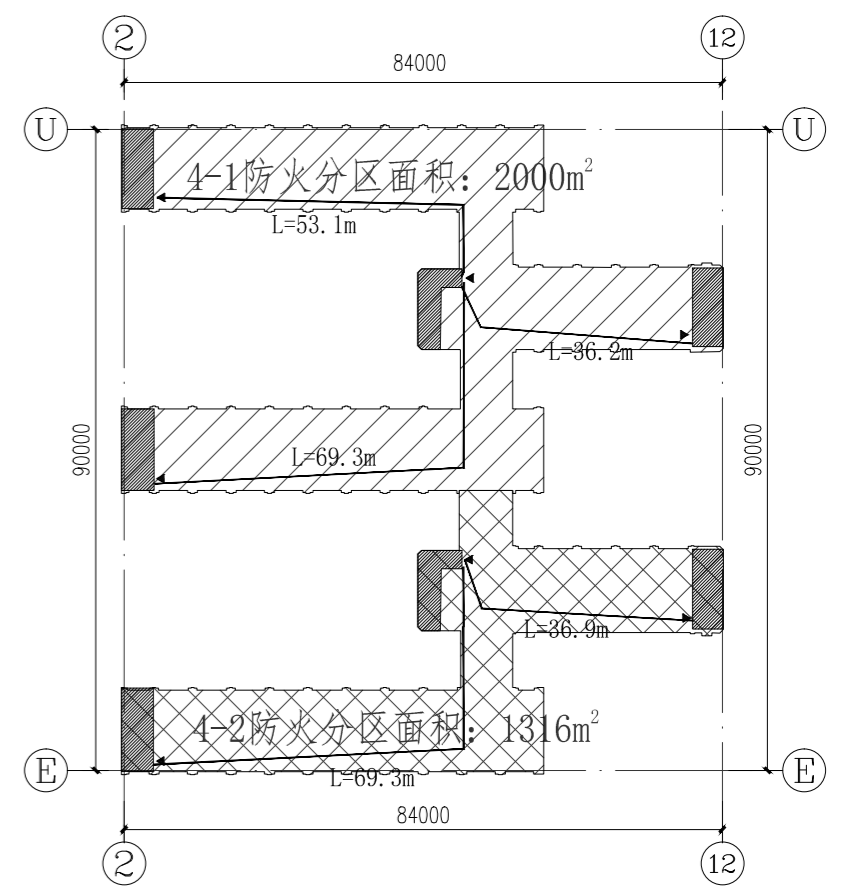
防火分区示意图
