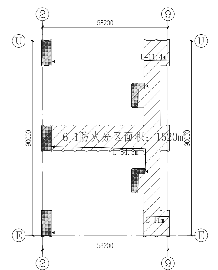
防火分区示意图
