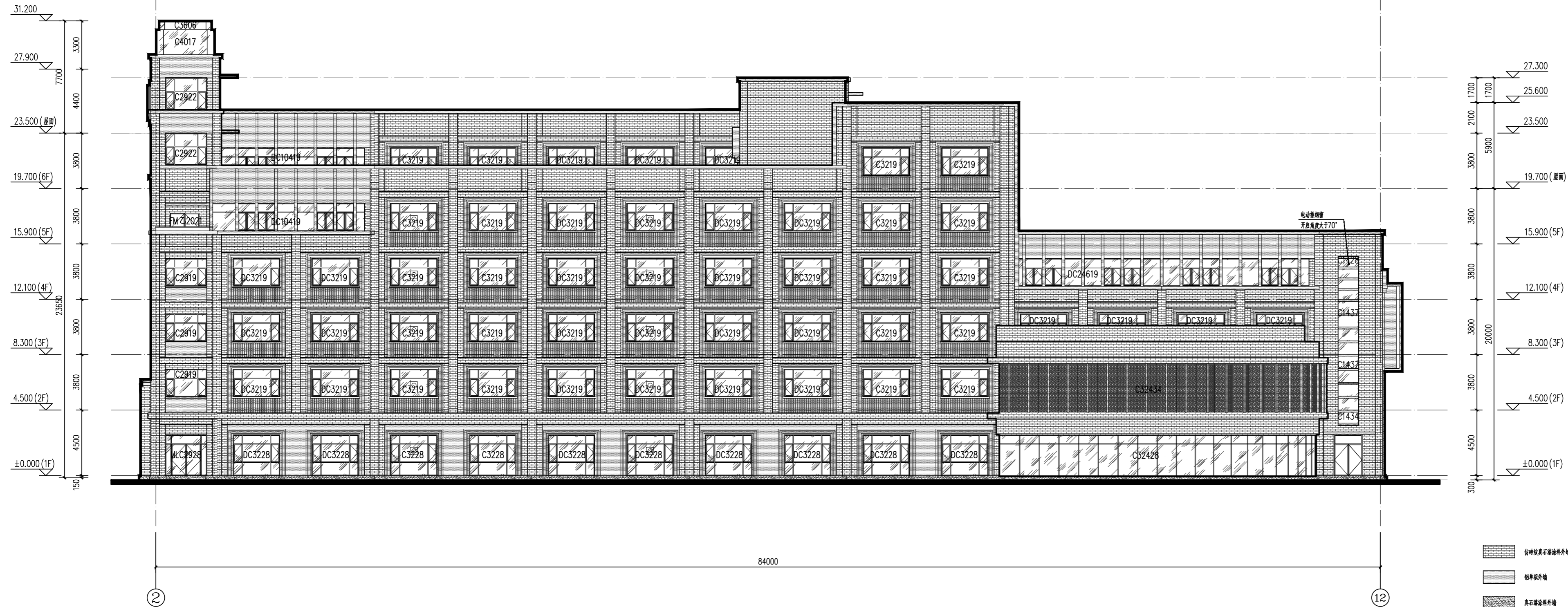
②-⑫立面图 1:150
