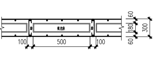
现浇空心板单元示意图
