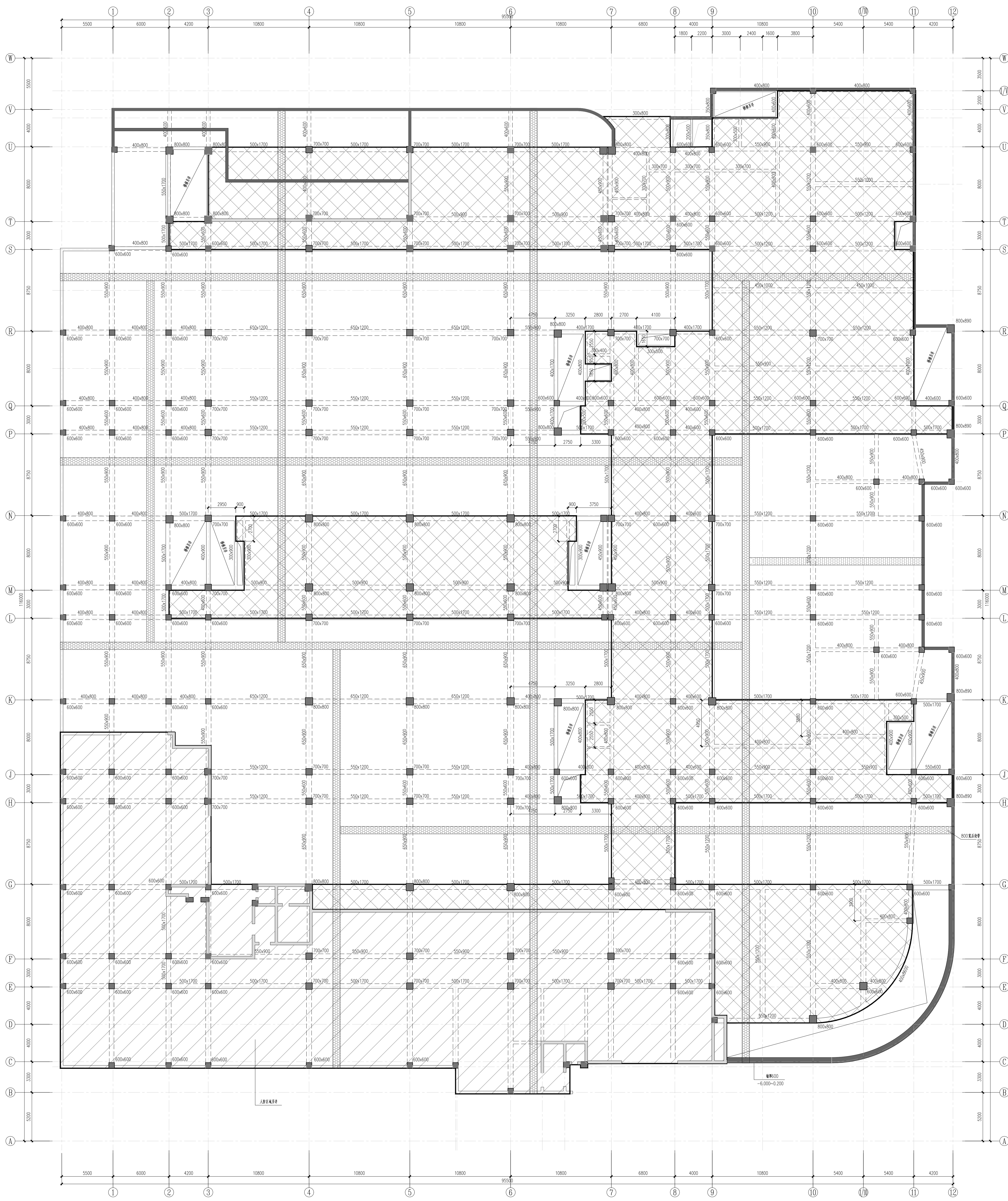
地下室顶板结构平面布置图
