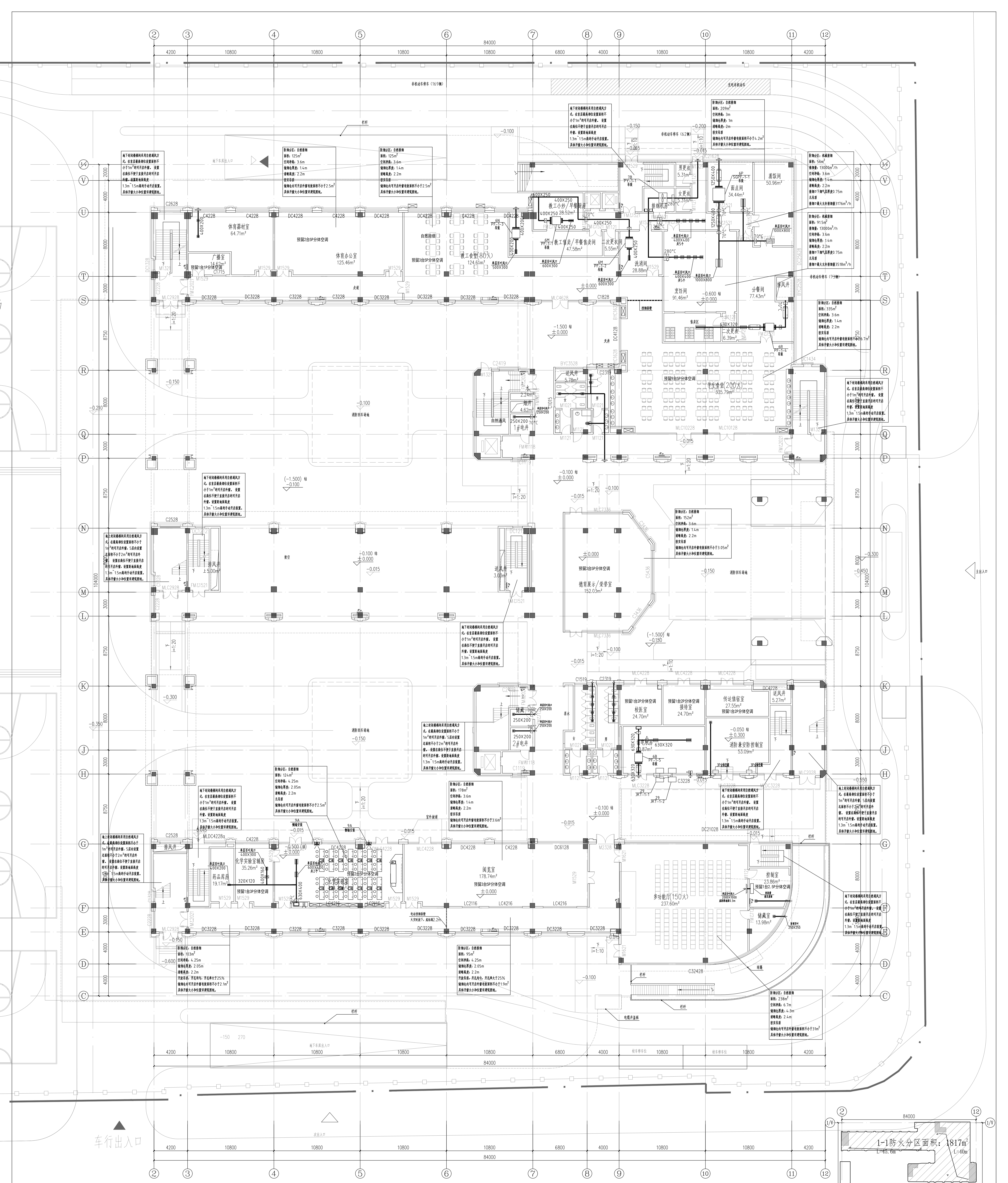
一层空调通风防排烟平面图 1:150
